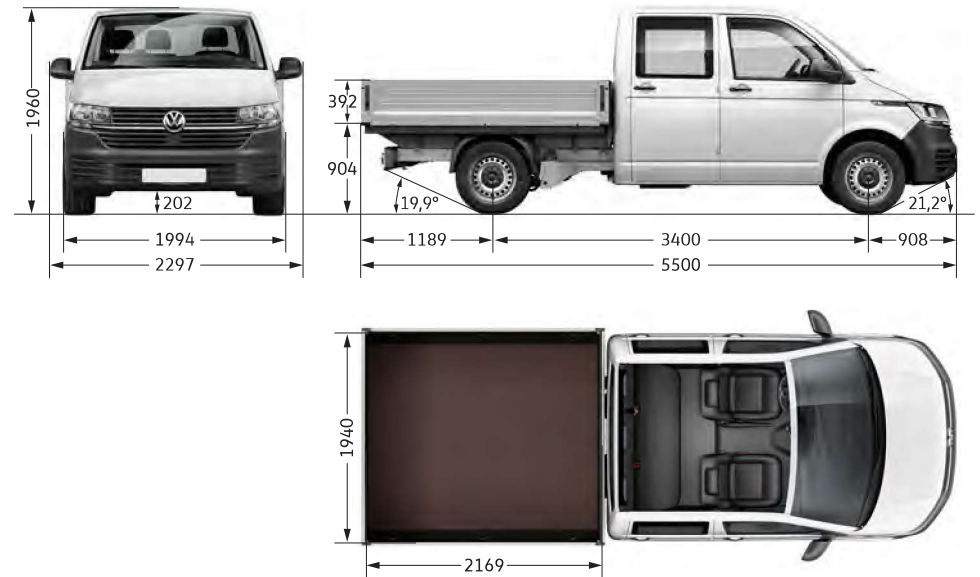
Transporter 6.1 Pritschenwagen mit langem Radstand und Doppelkabine
