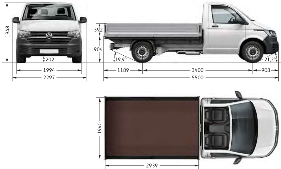
Transporter 6.1 Pritschenwagen mit langem Radstand und Einzelkabine
